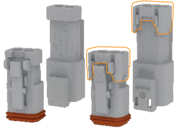
DT 焊接式后盖连接器
