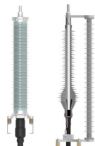
最大 145 kV の常温収縮ドライタイプ結線
