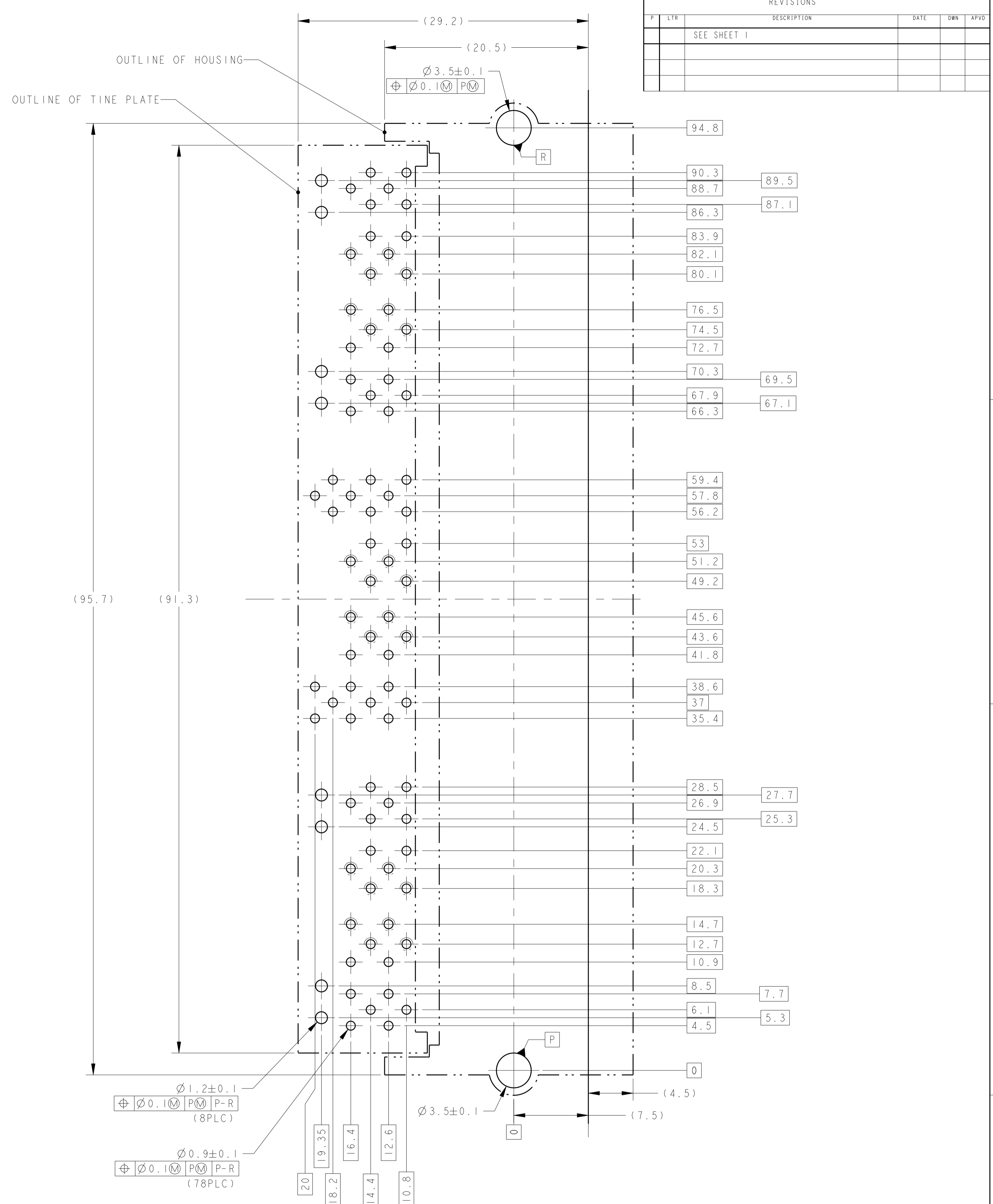
FIG. 3 RECOMMEND DIMENSION FOR P.C.B
