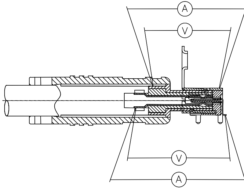
図 1 コンタクト及びシェル抵抗測定点
