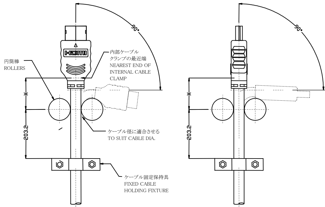
図 3 ケーブル屈曲試験方法
