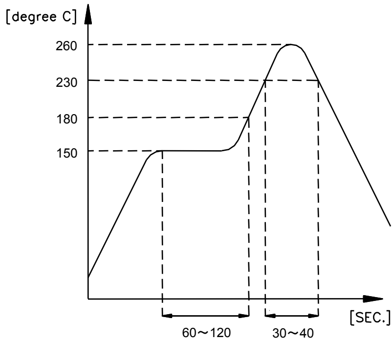
図 4 リフロー温度プロファイル
