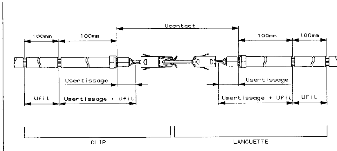
Figure 1 Montage de mesure des résistances de sertissage et du contact
