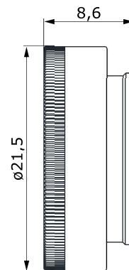
Hauptabmessungen Schirmelement
