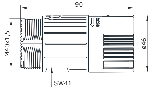
Hauptabmessungen Stecker
