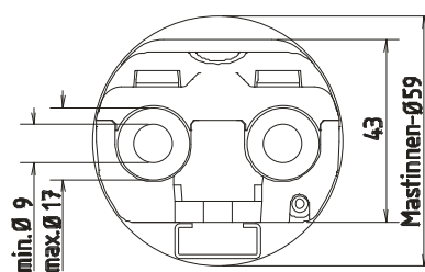
Kabelzugang
