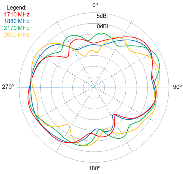
Elevation 1
