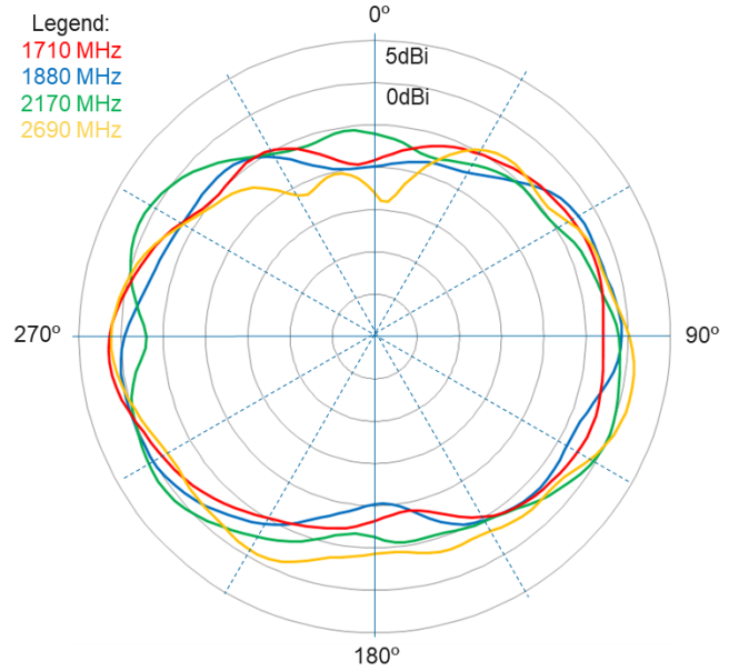
Elevation 2
