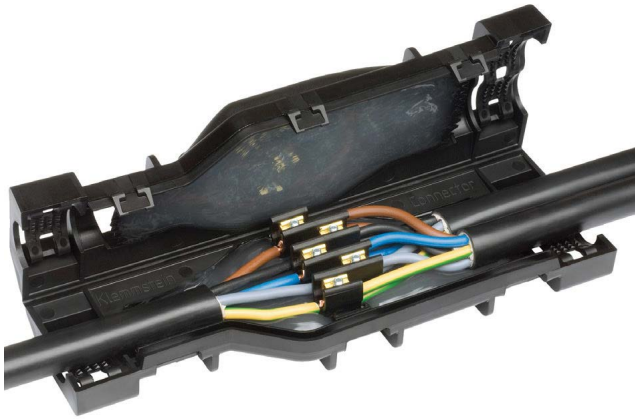
RayGel Plus 2 Muffe mit installiertem Verbinderblock
