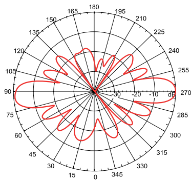
E-PLANE 2.45 GHz
