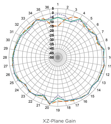
XZ-Plane Gain
