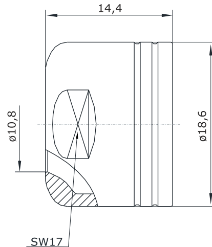
Hauptabmessungen Klemmring
