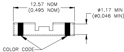
4) CRIMP, Qty/kit: 2
