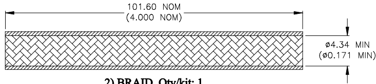
2) BRAID, Qty/kit: 1
