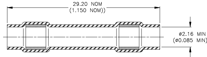
5) SEALING SLEEVE, Qty/kit: 2
