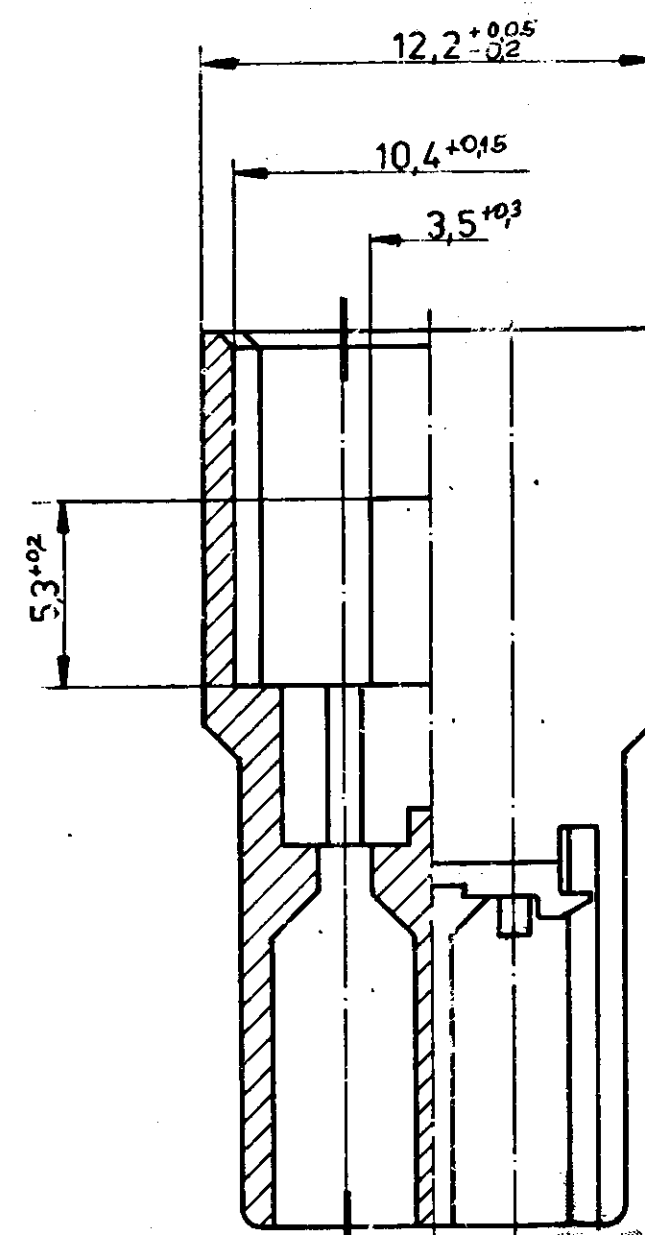
Schnitt C-D
