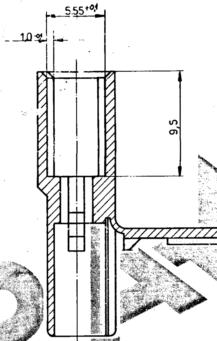
Schnitt A-B
