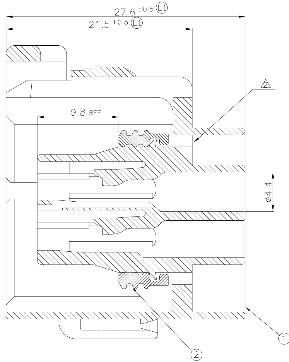
SECT A-A
