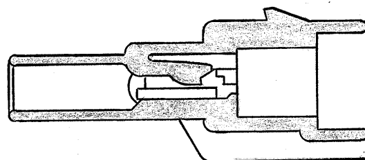
断面 A-A
