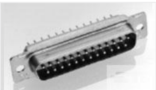
TE 产品编号211635-4 HD109 25 POS GMT ASY RCPT
