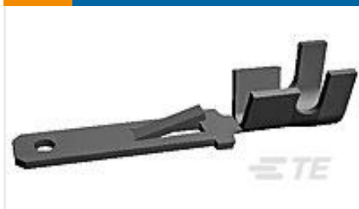
TE 产品编号160859-4 FF 250 TAB 20-17 AWG .016 TPPB
