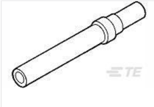
TE 产品编号205090-1 HD 20 SOCKET CONTACT
