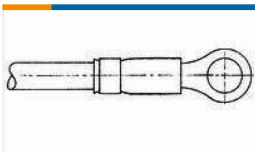
TE 产品编号131149-1 TERMINAL, RT, STRATO, POST INS, 8
