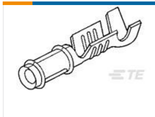
TE 产品编号60789-8 .058 DIA RECEPTACLE LP 20-24 GPBECU
