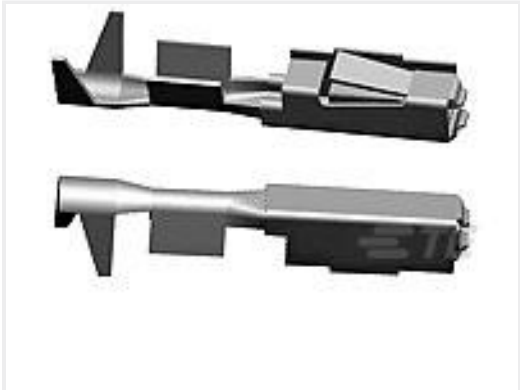
TE 产品编号5-928999-5 MQS0,63 Au rec LL unseal. >0,2-0,35
