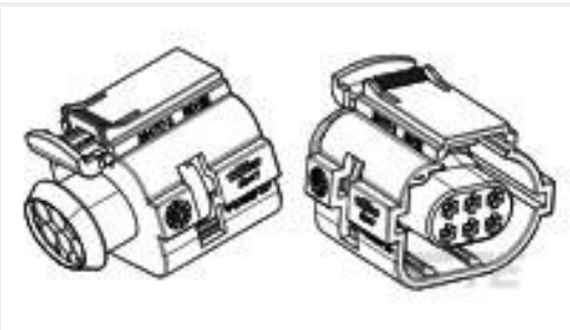
TE 产品编号284716-4 6 P. REC CONN X UEGO CONN
