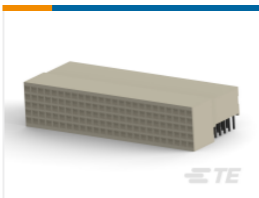
TE 产品编号5646446-1 HM 插座连接器：传统背板，共面， 2mm
