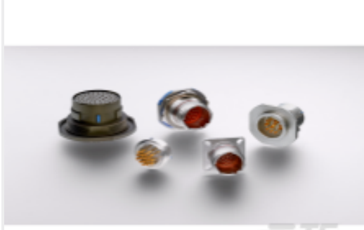
TE 产品编号 YDTS23H25-04SEV001 HERM RECP
