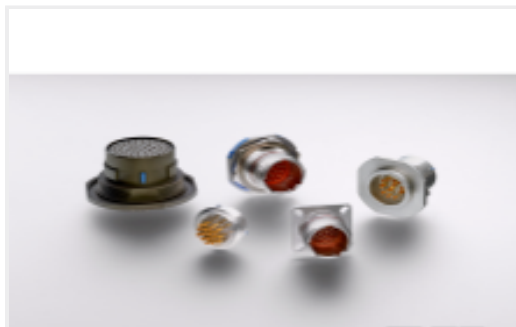
TE 产品编号 YDTS23N11-98CNV001 HERM RECP
