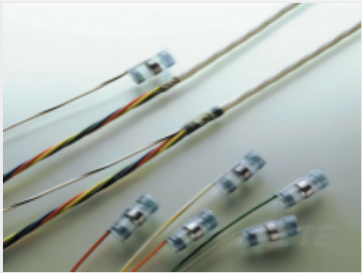
TE 产品编号439220-000 ST18-3-55-22-9
