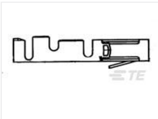
TE 产品编号87667-1 MOD IV RECP LP
