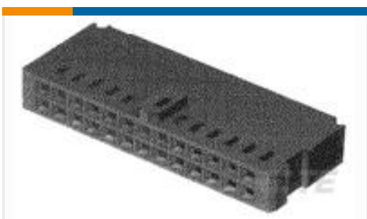
TE 产品编号1-102387-0 50 MODIV HSG COMP DR .100 POL
