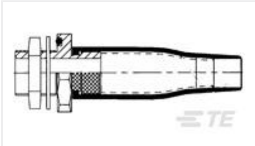
TE 产品编号511381-000 TCFS-16-62C-020-100CH
