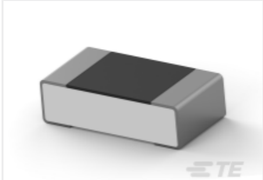
TE 产品编号6-2176369-0 RQ 0603 165R 0.1% 10PPM 5K RL
