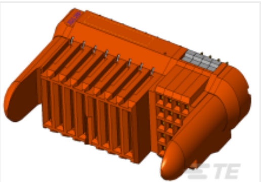
TE 产品编号1892787-9 Assy Vert MINIPAK HDL Rcpt 20s
