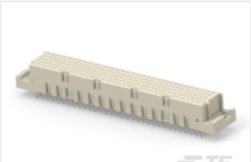
TE 产品编号284314-E STVE 160 F ABCDE VVVV 7-00 TL 4,0 * 247
