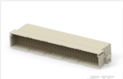
TE 产品编号364918-E STVCD 128 M ABCD VVV 4-00 0606 * * 247
