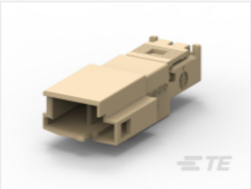
TE 产品编号2203701-1 2POS, MCON 1.2 CB TAB 2p TL UNSEALED
