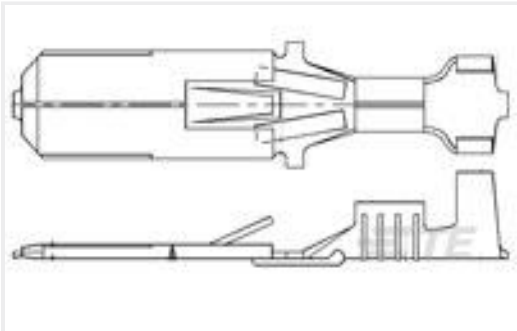
TE 产品编号280081-2 FF 250 TAB 0.8-2MM2 TPBR
