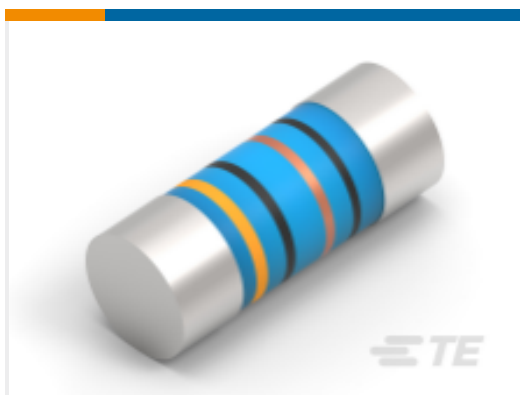
TE 产品编号1-2176335-5 MELF SMA-A 160R 1% 50PPM 0102 0.3 W
