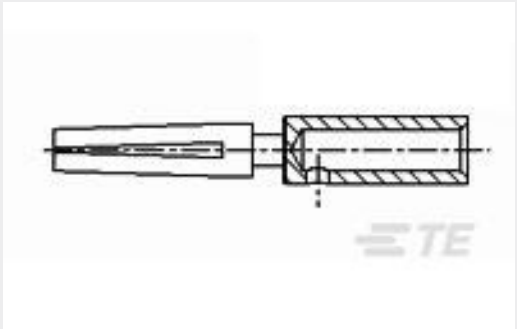
TE 产品编号5-1437720-6 T01-CRIMP-S03
