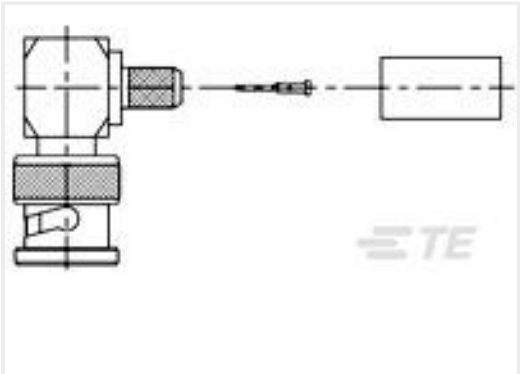
TE 产品编号1-1337440-0 BNC R/A Plg Hex 75Ohm Silver Pltd RG179B
