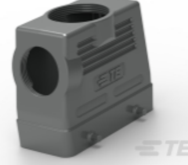
TE 产品编号 T1190162940-000 H16B-TGH/TSH-M40/PG29
