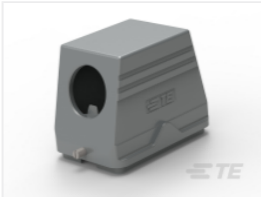
TE 产品编号 T1310480142-000 H48B-TS-RO-PG42
