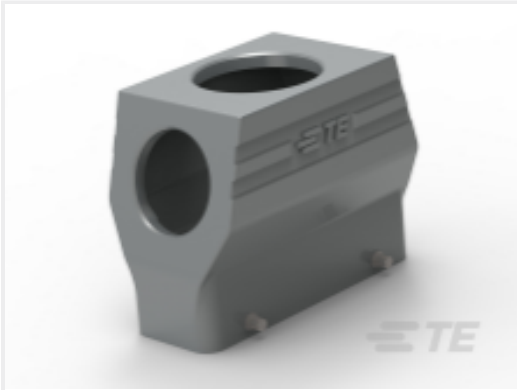
TE 产品编号T1196245040-000 H24B-XWTG/TS-M40/M50
