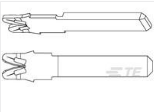
TE 产品编号4-1601051-2 031-113-014=TAB,118X032,STD SMZ
