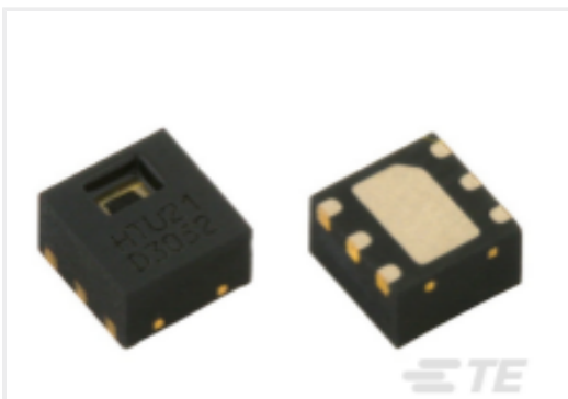
TE 产品编号HPP845E031R4 I.C 21D RH/T B400
