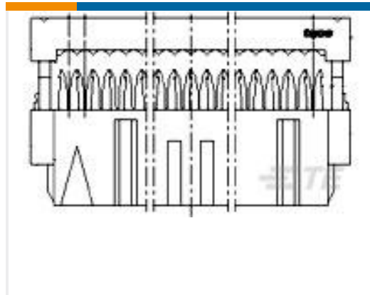
TE 产品编号2-215882-0 20 WAY GREY MK II RECP
