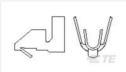
TE 产品编号3-770565-1 MINI AMP-IN 22-18 AWG SN/BRASS LF
