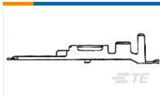
TE 产品编号172777-1 MIC MARE-2 TAB CONTACT
