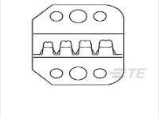
TE 产品编号90575-2 SDE UMNL 20-14 AWG DIE
