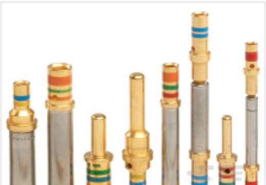
TE 产品编号4160-204-1631L CONT PIN
