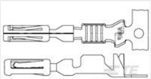
TE 产品编号770520-3 AMPSEAL,TERMINAL,GOLD PLATE, 16-20AWG WIR
